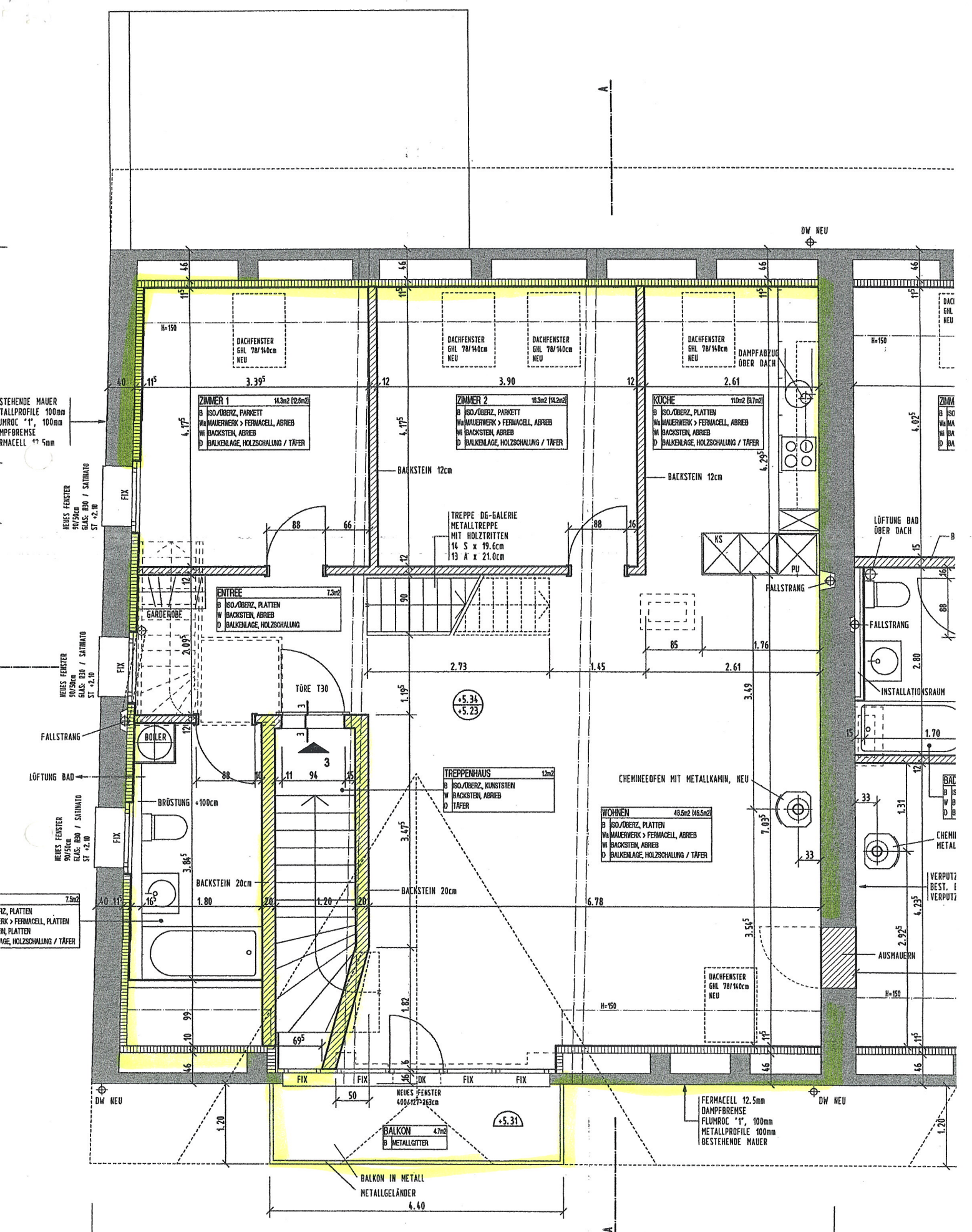
APPARTEMENT 3 4 1/2 CH. NF = 173.2 m² (128.1m² über 1.50m Höhe) MAISON "A" SGF = 207.9m² (147.6m² über 1.50m Höhe)
